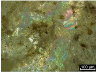
Optische Mikroskopie der Oberfläche einer PET Flasche
