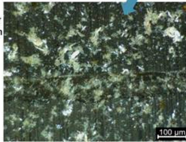
Optische Mikroskopie von PET Mikroplastik nach Auftragen der wässrigen Suspension auf einen geeigneten Träger.
